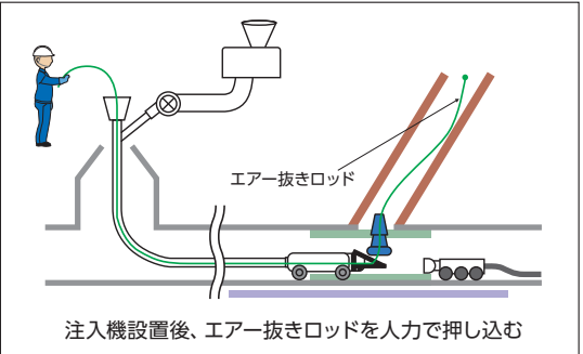
注入量確認測定、エア抜き設置
